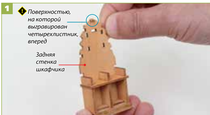
1 К нижней части шкафчика, собранной в выпуске 35, при помощи клея для дерева прикрепите заднюю стенку.
